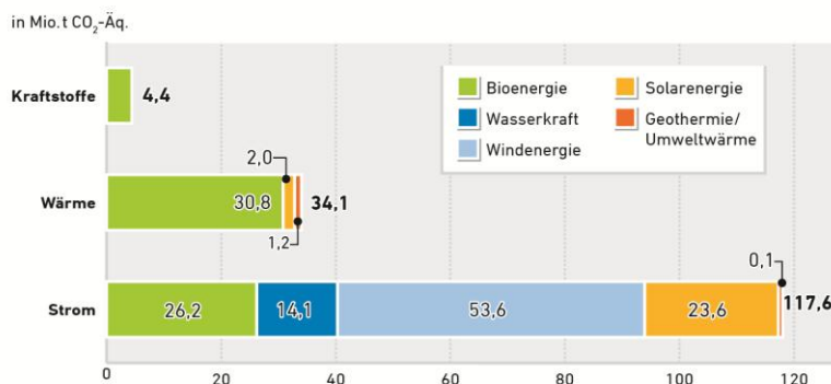
Vermiedene Treibhausgas-Emissionen durch die Nutzung Erneuerbarer Energien in Deutschland 2015 Erneuerbare Energien vermieden 2015 rund 156 Mio. Tonnen CO 2 -Äquivalente.
